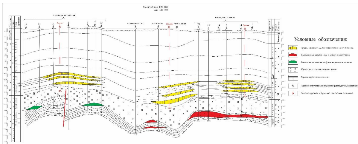
Рис. 3. Геологический профиль по линии структур Уртабулак-Султошох-Сардоб-Чистон-Зеварды
