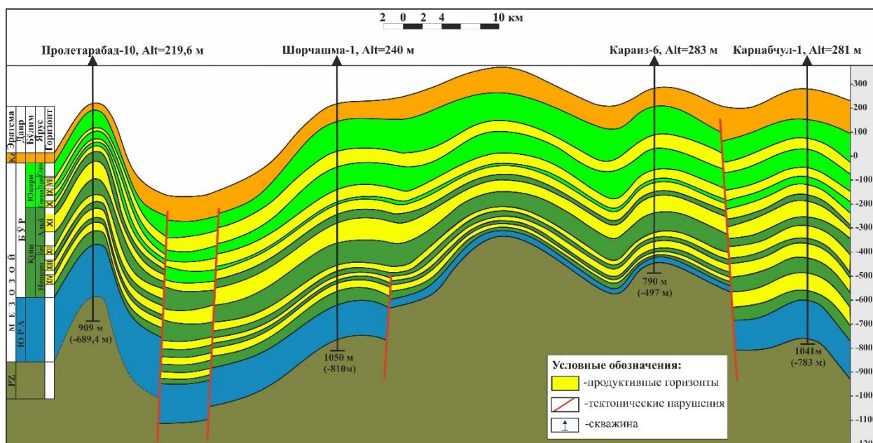
Рис. 2. Геологический профиль по линии площадей Пролетарабад-Шорчаишма-Караиз-Карнабчуль (по материалам М.С. Махмудовой, 2026 г.)
