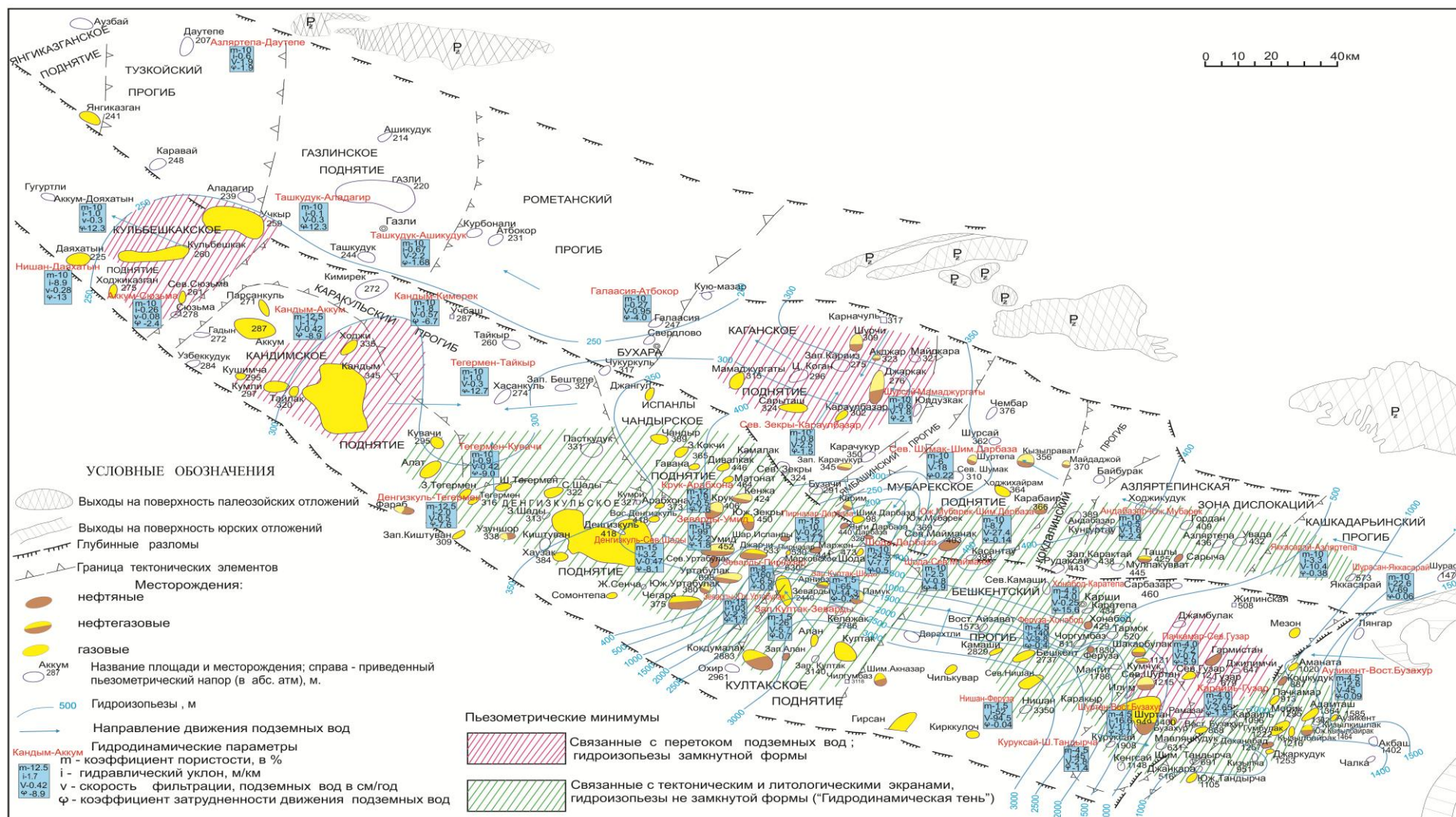
Рис. 5. Схематическая гидродинамическая (гидроизопьез) карта нижнемеловых отложений Бухаро-Хивинского нефтегазоносного региона
