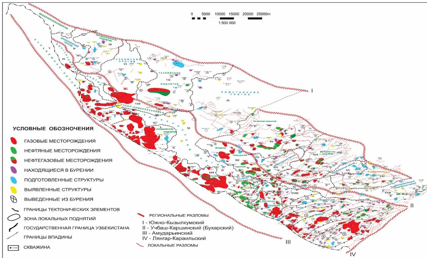
Рис. 1. Схематическая тектоническая карта Бухаро-Хивинского региона с размещением месторождений нефти и газа и перспективных площадей
