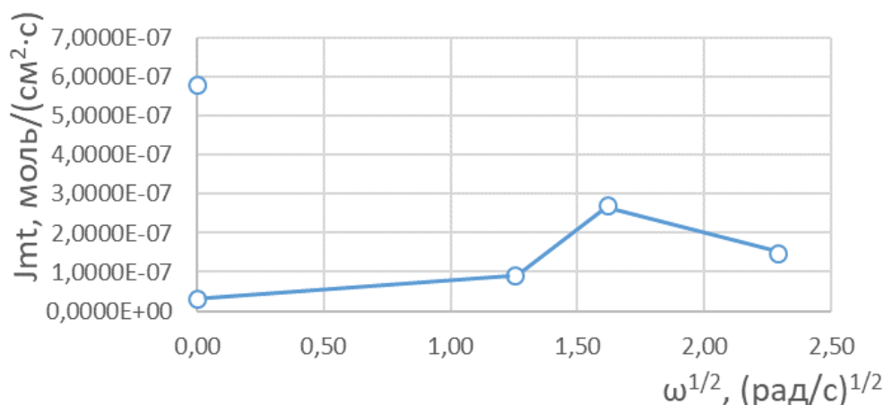
Рис. 2. Фактическая зависимость скорости реакции от корня квадратного угловой скорости вращения диска для керна с КС
