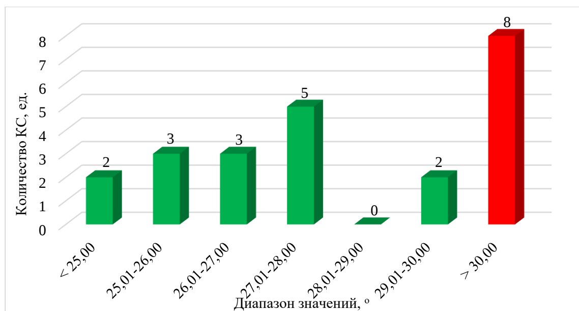
Рис. 9. Распределение КС для ОПЗ карбонатных коллекторов по их предельным значениям угла смачивания
