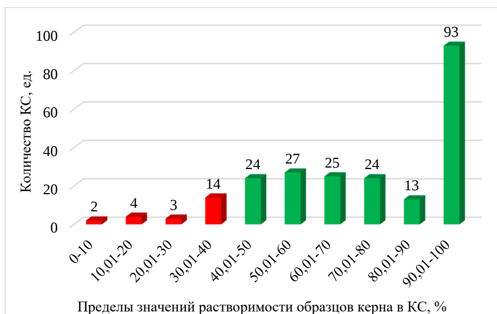
Рис. 5. Распределение КС для матричных и селективных ОПЗ карбонатных коллекторов по их предельным значениям растворимости образцов керн
