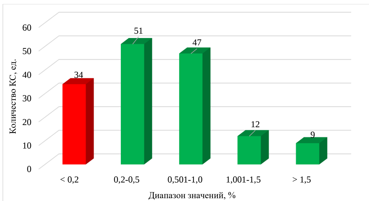
Рис. 6. Распределение КС для ОПЗ терригенных коллекторов по их предельным значениям растворимости образцов керна
