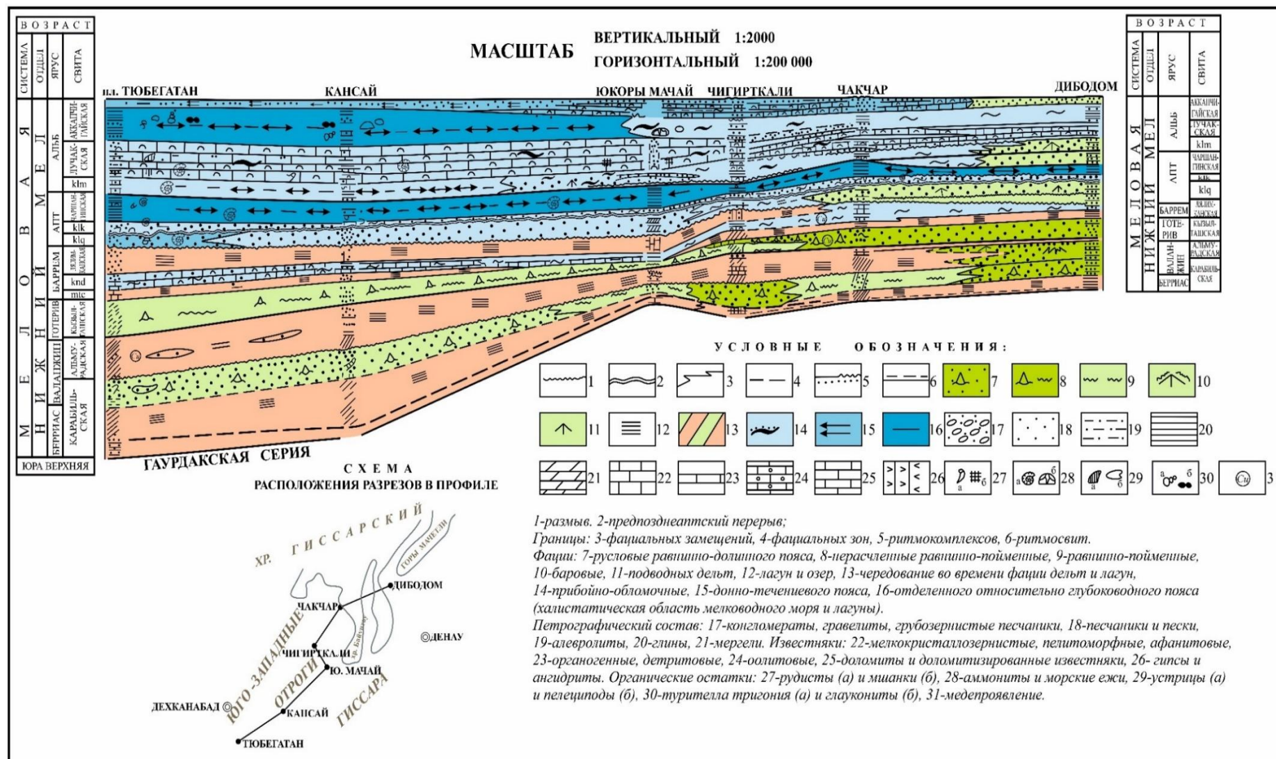
Рис. 2. Литолого-фациальный профиль отложений нижнего мела центральной части Юго-Западного Гиссара по линии Тюбегатан-Кансай-Юкоры Мачай-Чигирткали-Чакчар-Дибодом (III-III)
