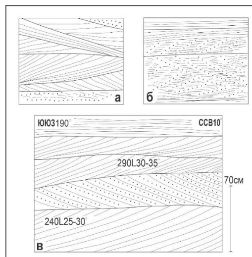
Рис. 7. Косая перекрестная (а), косоволнистая типы ряби мелководья (б) и косая «ёлочковидная» (в) сло́йчатость причудливой морфологии кирпично- красных и вышнево-бурых песчаников и алевролитов кызылташской свиты (готерив)
