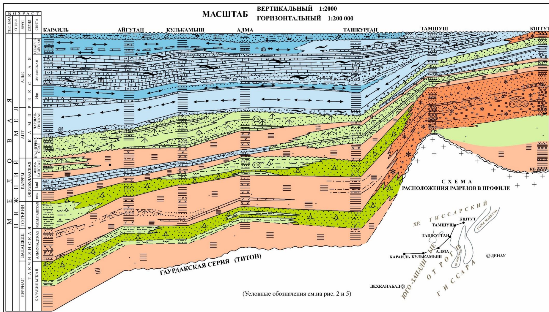
Рис. 4. Литолого-фациальный профиль нижнемеловых отложений Юго-Западного Гиссара по линии Караиль-Айгутан-Кулькамьш-Алма-Ташкурган-Тамшуш-Китут (V-V)
