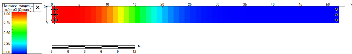
Рис. 2. Модель, состоящая из 50 ячеек размером 1 м между скважинами
